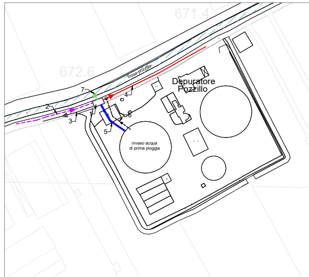
SCHEMA IDRAULICO
